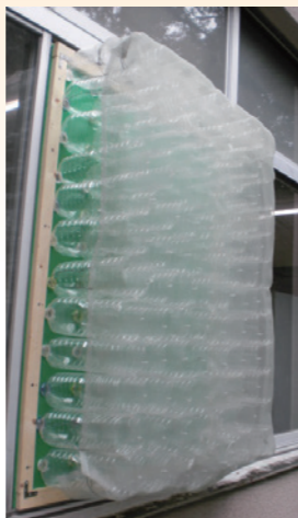
作品名 ペットボトルエコクーラー 製作者 愛知県立岡崎工業高等学校 機械デザイン科課題研究班
